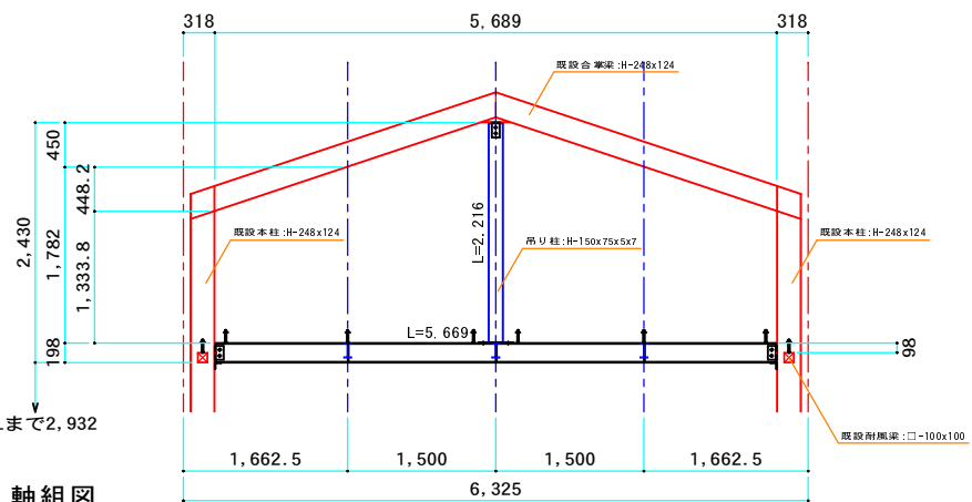
軸組図 S=1/60 (A3)
