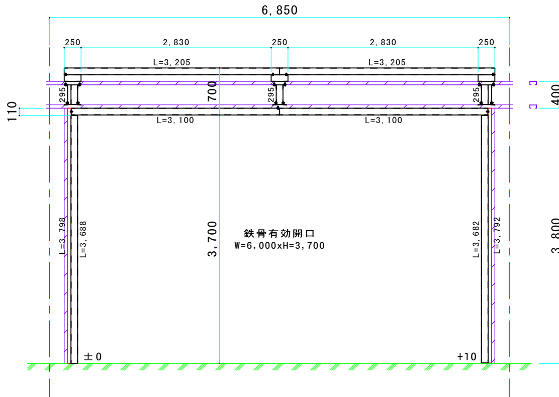
立面図 S=1/20
