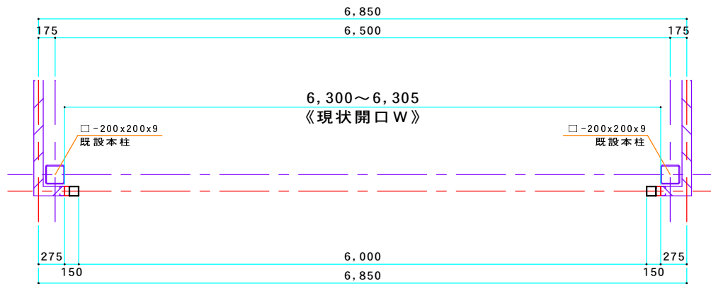
平面図 S=1/20
